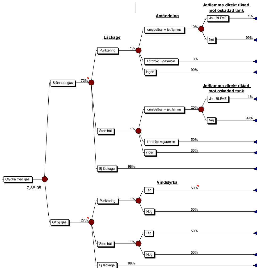
Figur D.4. Händelsetråd för farligt gods-olycka med gas i lasten.
