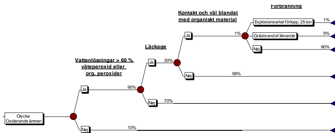
Figur D.6. Händelsetråd för farligt gods-olycka med oxiderande ämnen i lasten.
