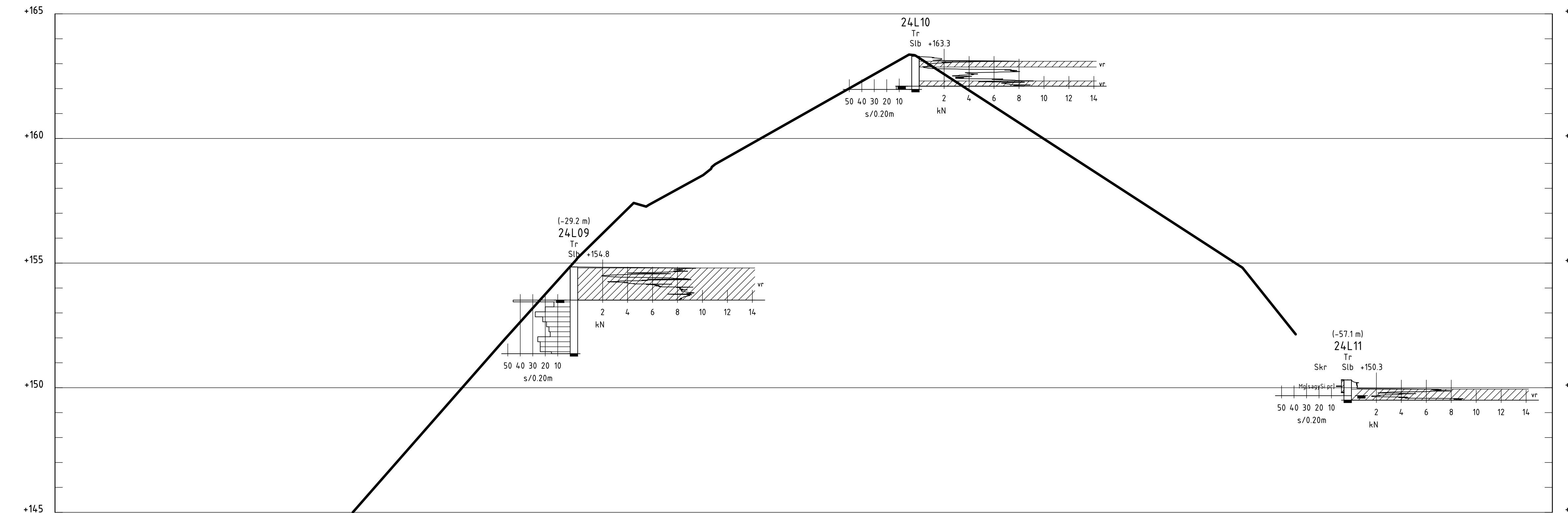
SEKTION D-D H 1: 100 L 1:1500
